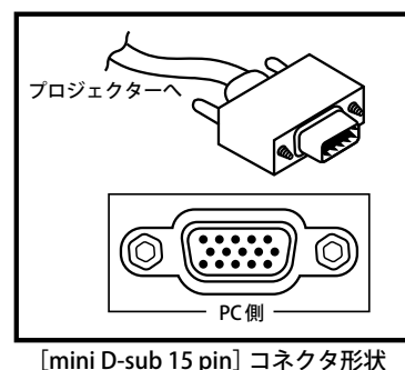
[mini D-sub 15 pin] コネクタ形状
